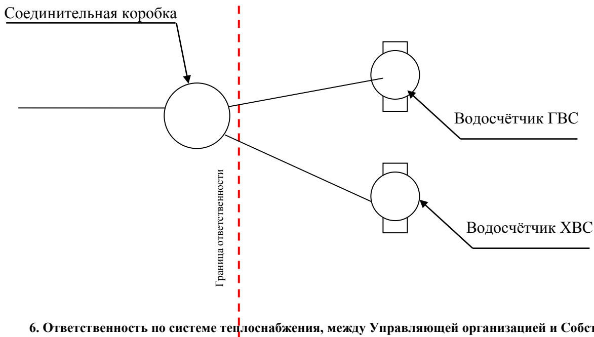
Схема № 5
